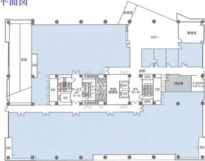
基準階平面図 (2-3F)
