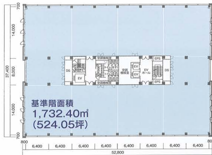
基準階平面図 (2-3F)
