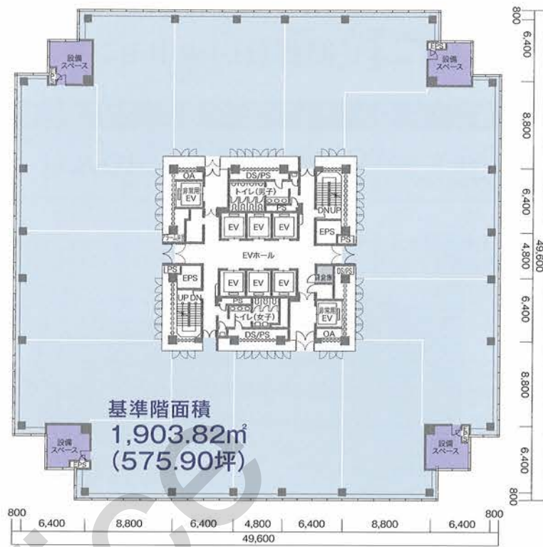
基準階平面図 (ウェストタワー3-10F)
