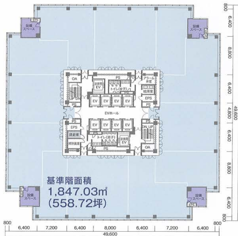
基準階平面図 (イーストタワー2-13F)
