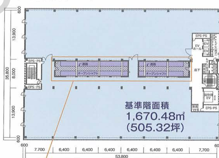
基準階平面図 (3-4F)
