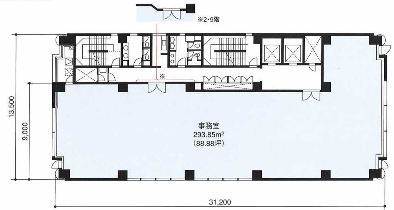
基準階平面図
