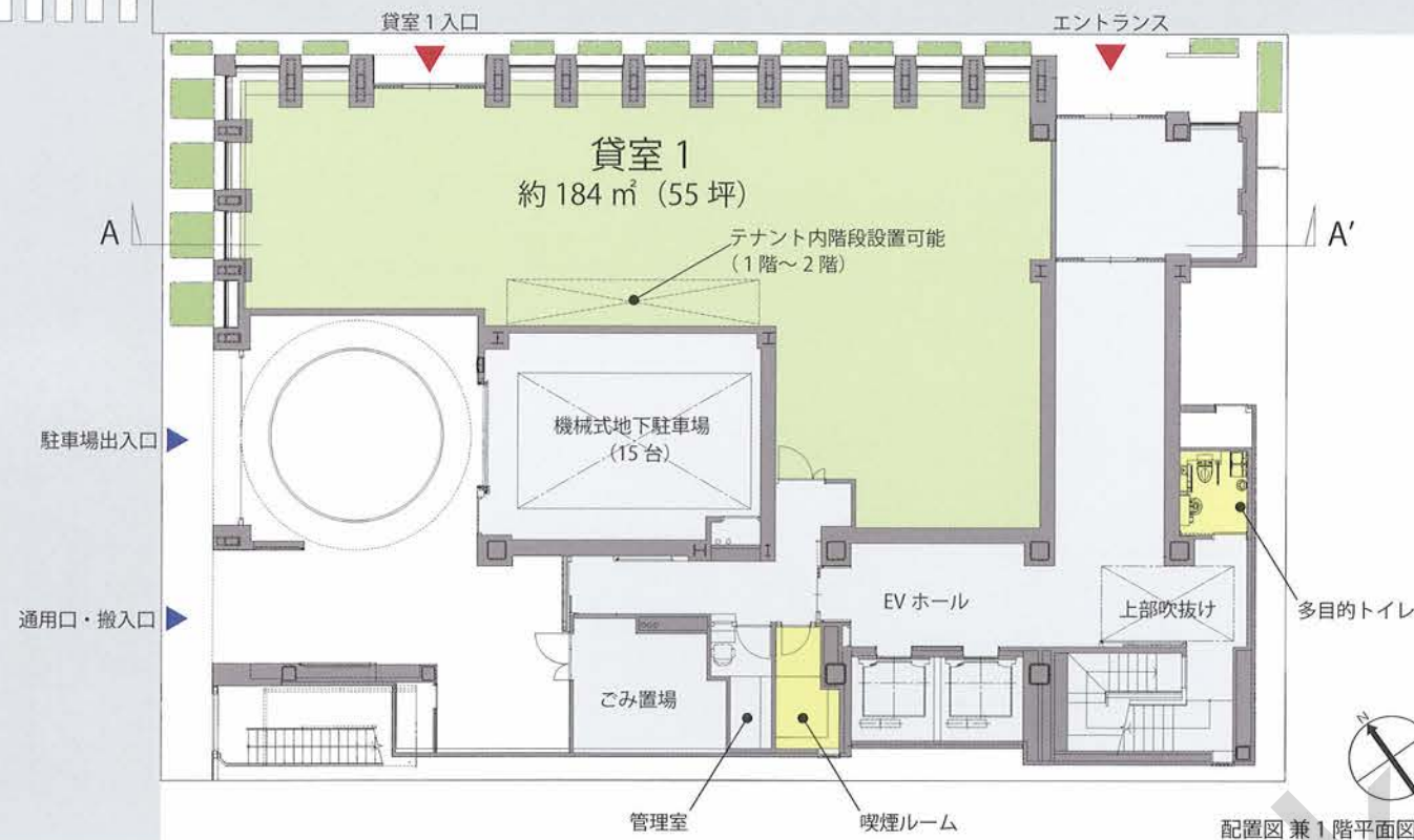
配置図 兼 1階平面図
