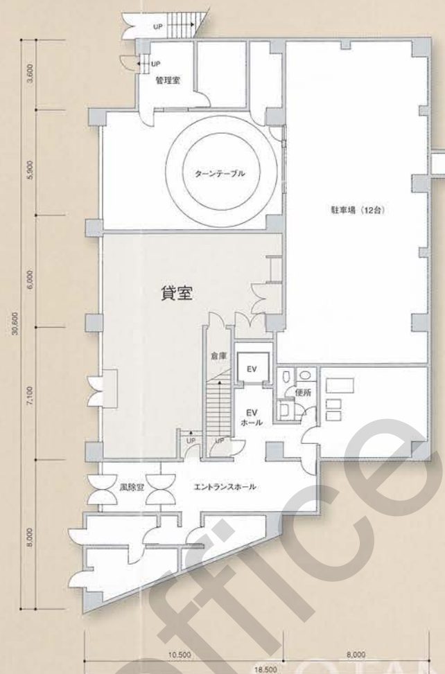
1階 平面図
