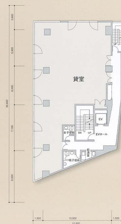
6~8階 平面図
