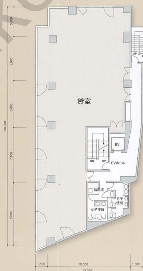
4・5階 平面図
