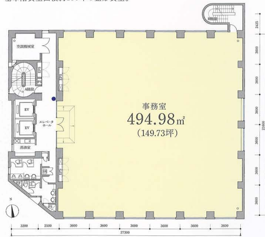
■ 基準階平面図(4階)
