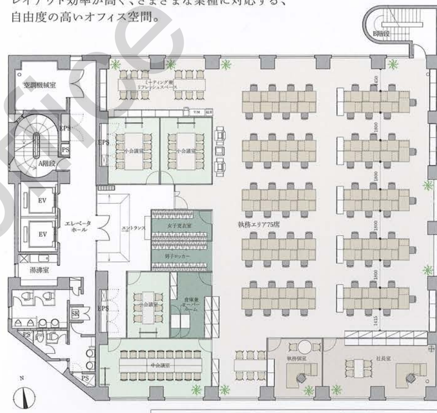
■ 基準階レイアウト
