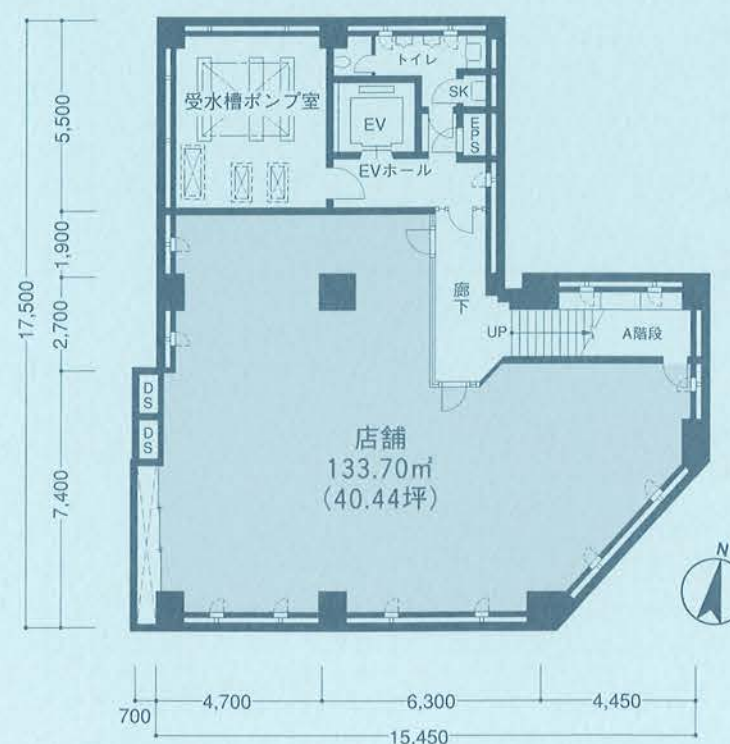
B1階平面図
