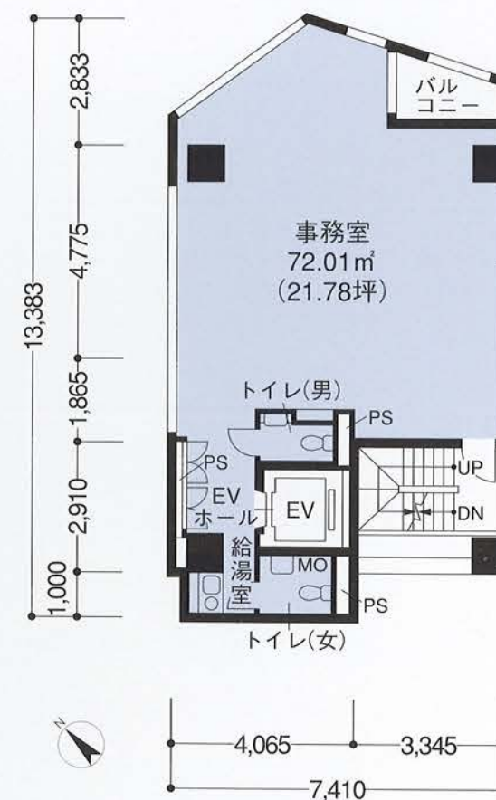
11・12階 平面図
