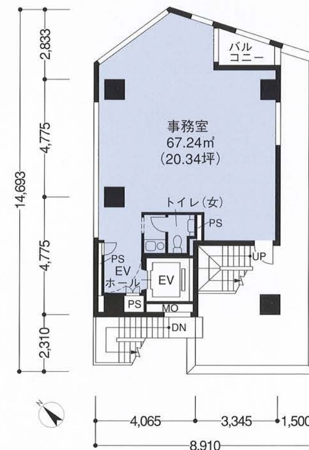
10階 平面図
