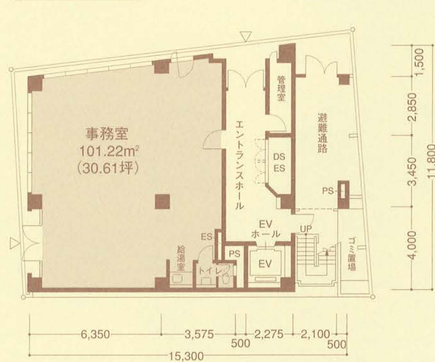
1階平面図
