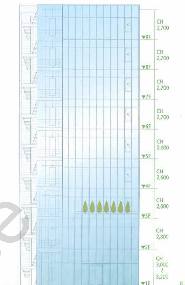
立面図(正面)
