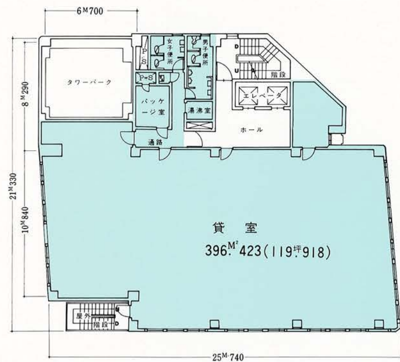
2～5階平面図
