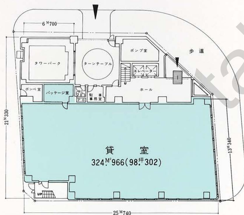
1 階平面図
