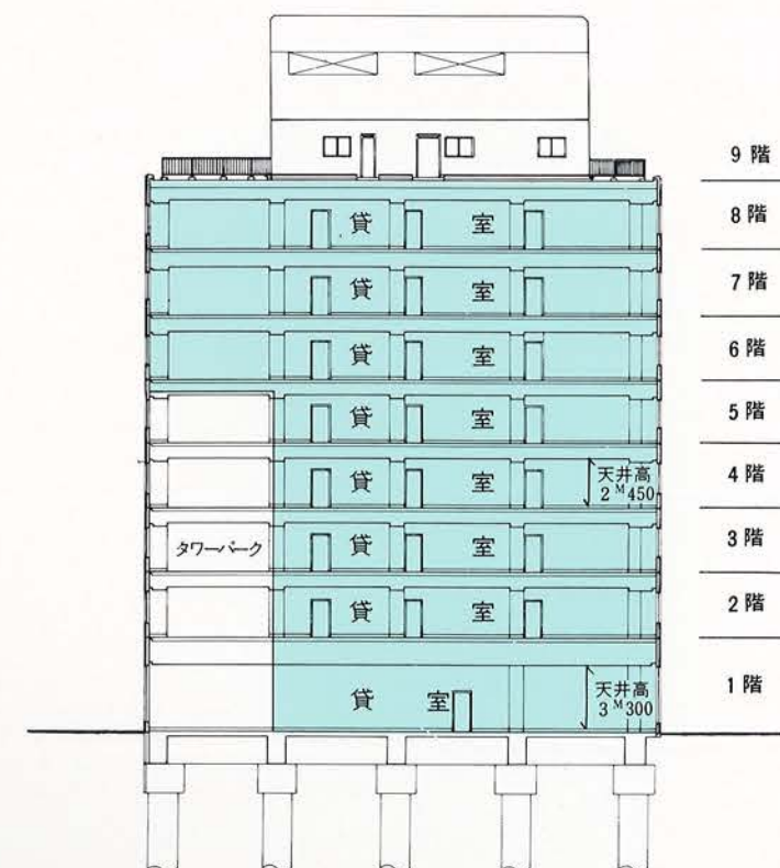
断面図
