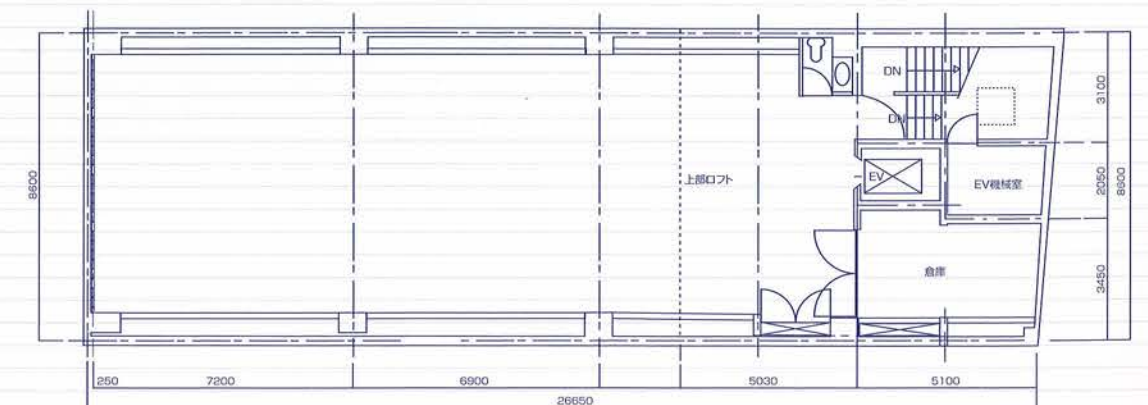
地階平面図
