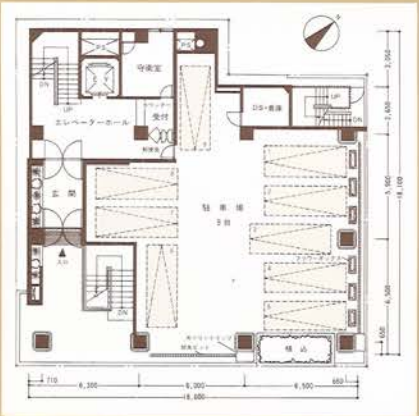
1階平面図
