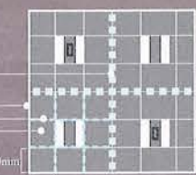
選択自在の天井パネル(点検口兼用) Ceiling panels can be freely positioned (and double as access panels). グリッドモジュールによる間仕切り位置 Partition placement for a grid module モジュールによる間仕切り位置 Partition placement for a single module ハーフモジュールによる間仕切り位置 Partition placement for a half module
