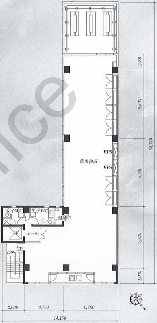
■3階～5階平面図
