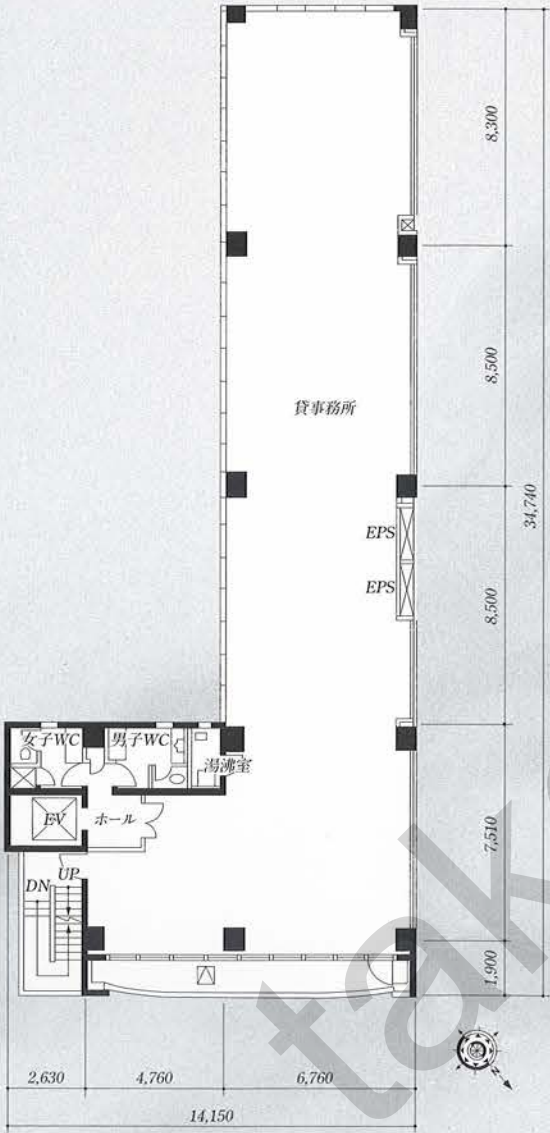
■2階平面図
