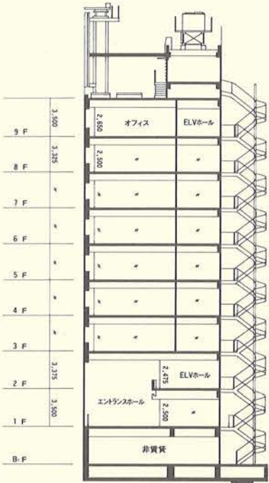
断面図
