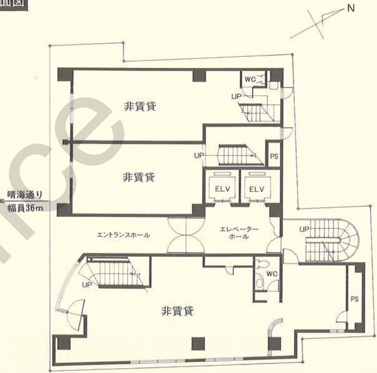
1階平面図
