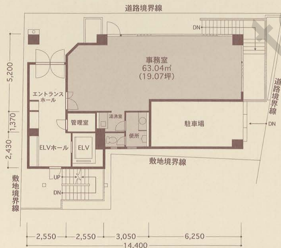
1F平面図
