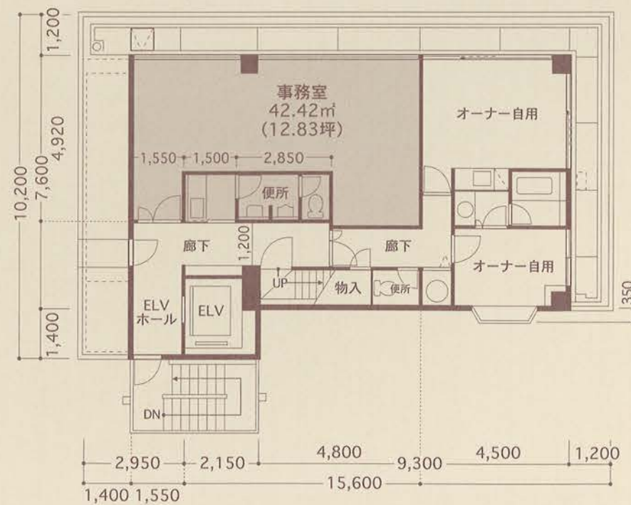
6F平面図
