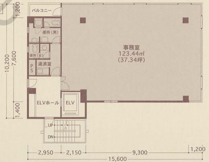
2F~5F平面図
