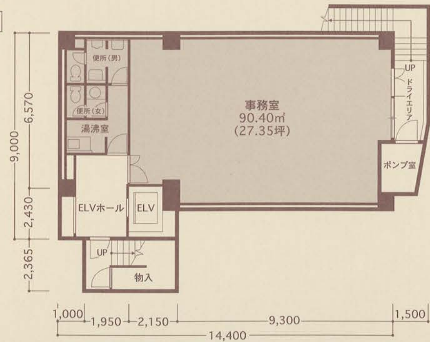
地階平面図
