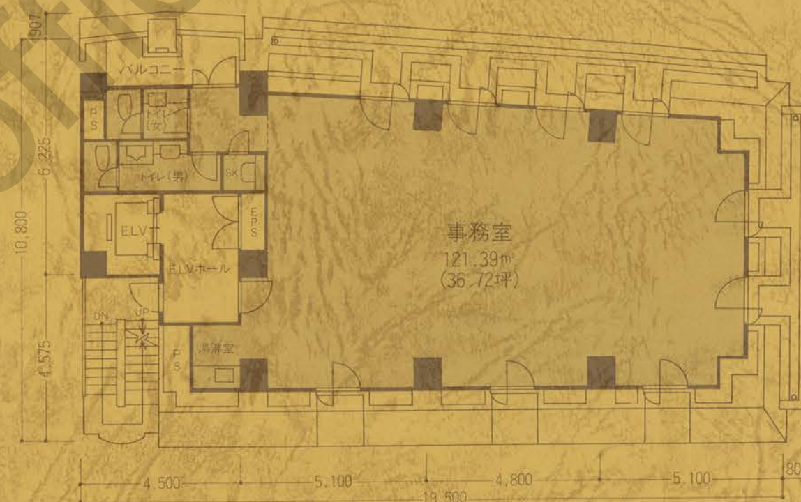
6階平面図
