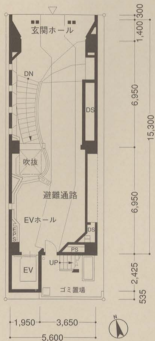
1階平面図
