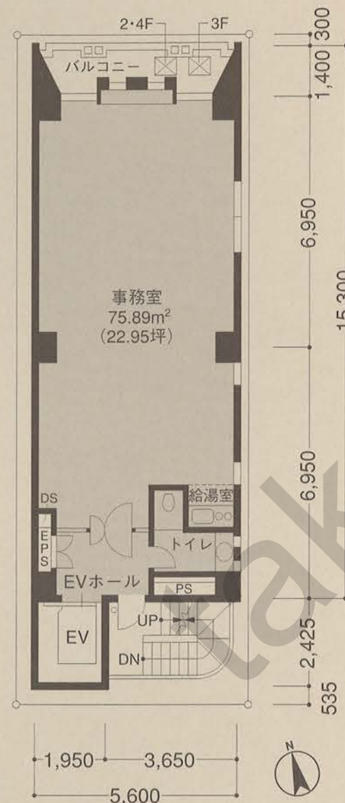
2～4階平面図
