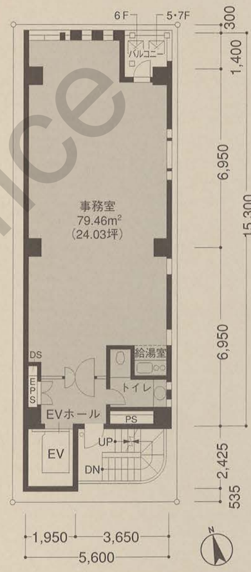
5～7階平面図
