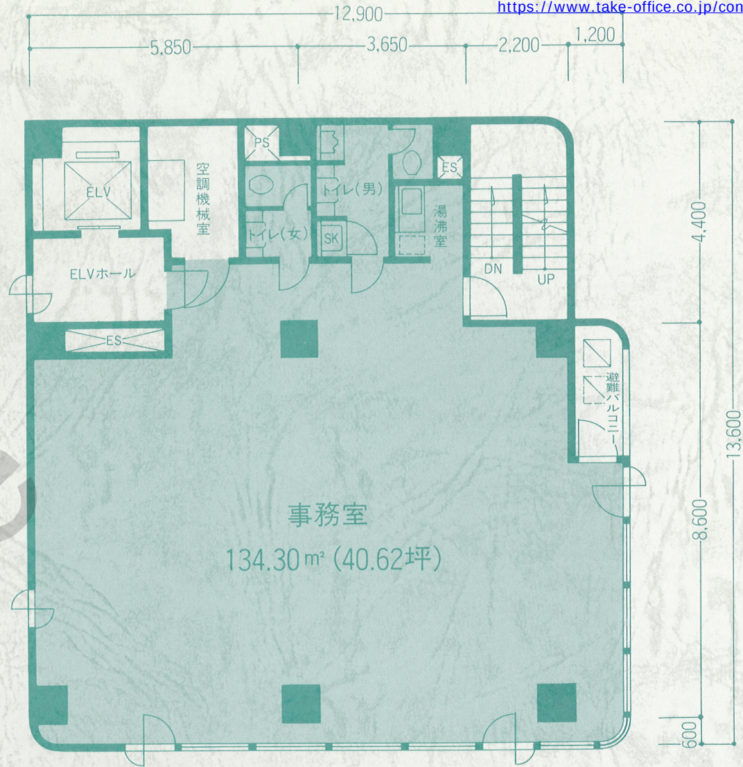
基準階平面図
