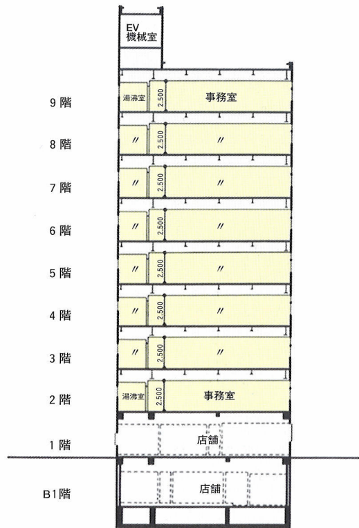
断面図
