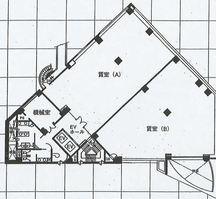
2階平面図
