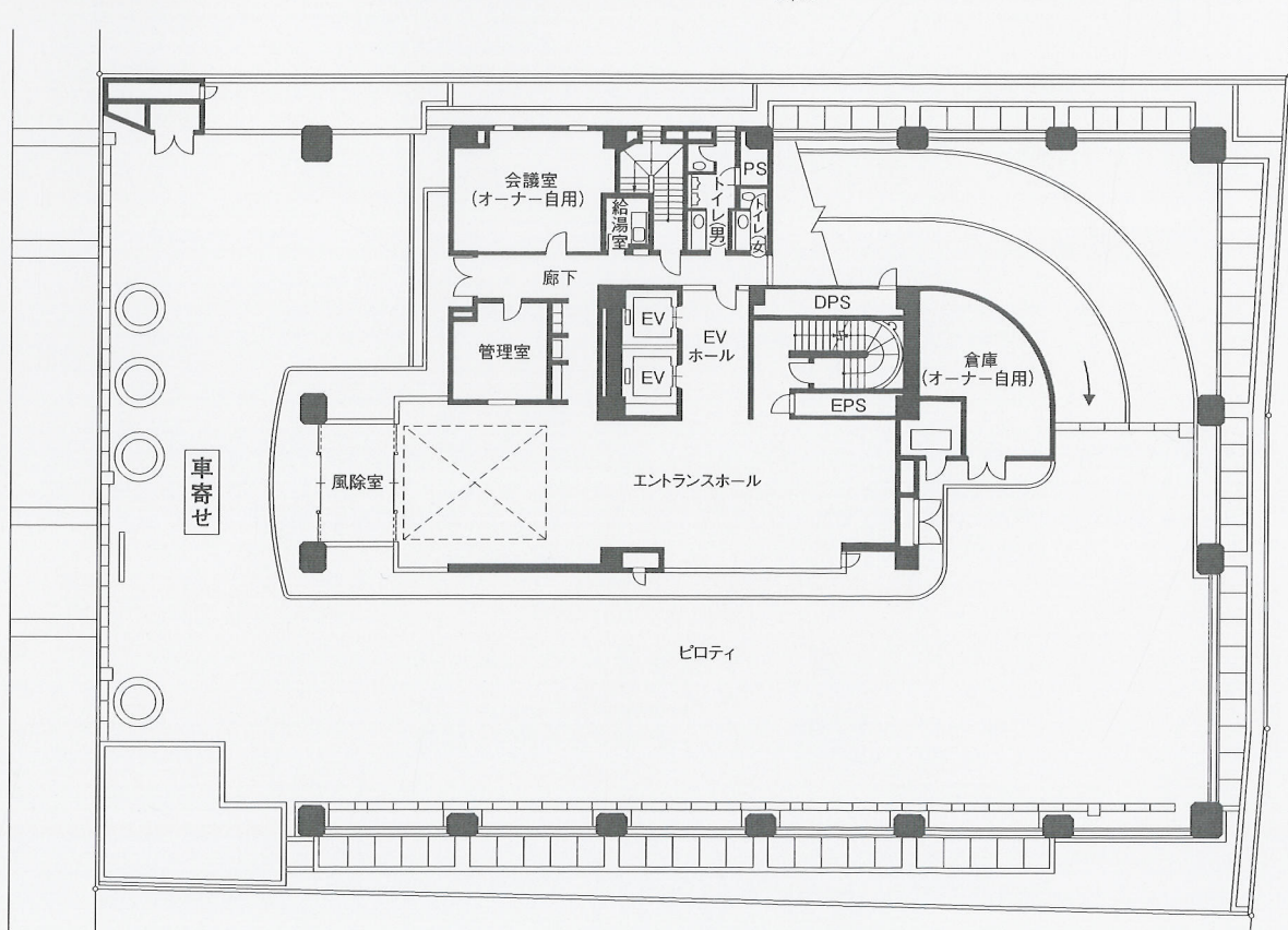
1階平面図
