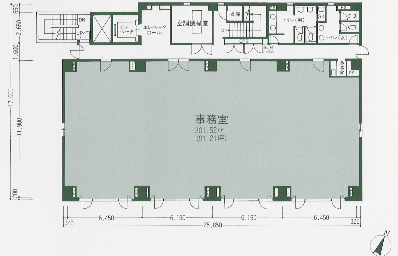
2・3階平面図
