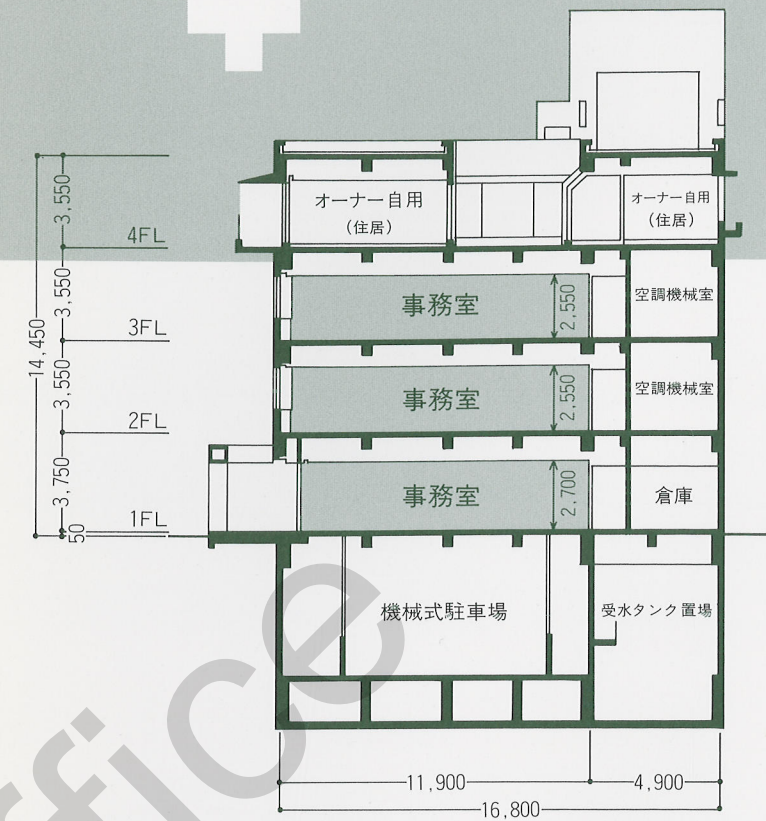
断面図
