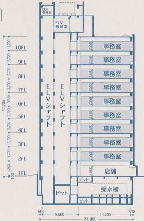
断面図
