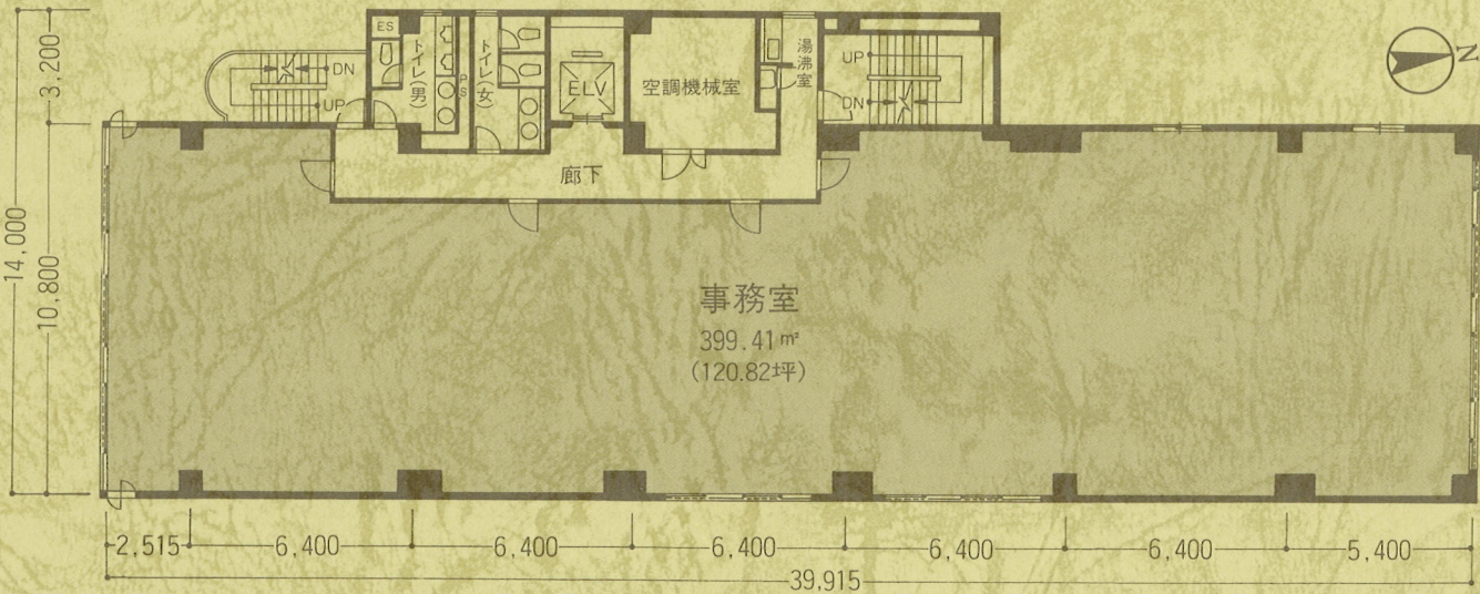
2～6階平面図
