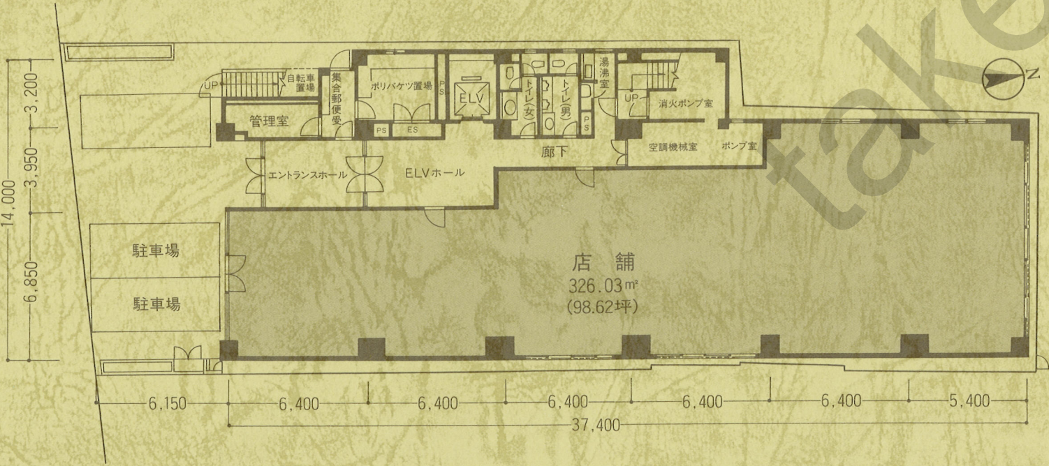
1階平面図
