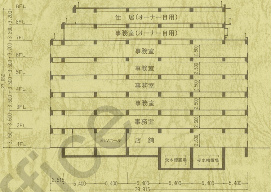
断面図
