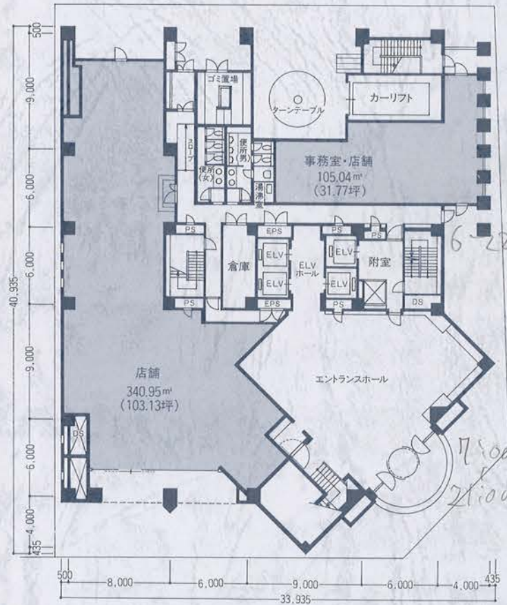
1階平面図
