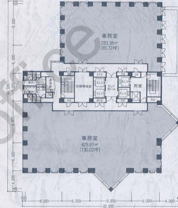
3階平面図
