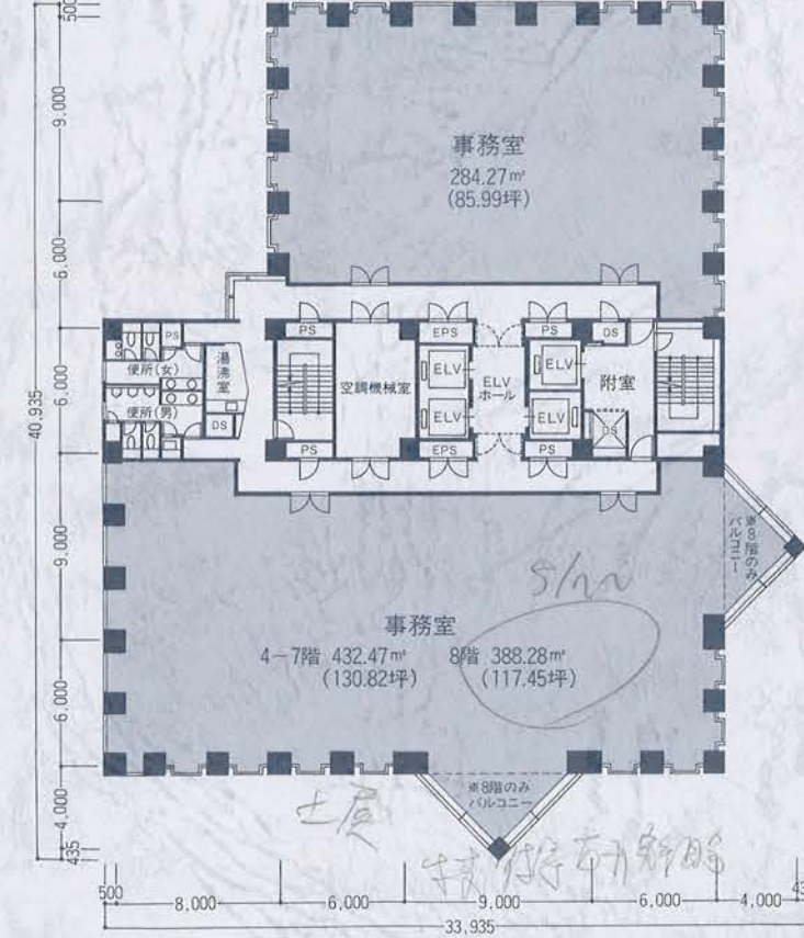
4～8階平面図
